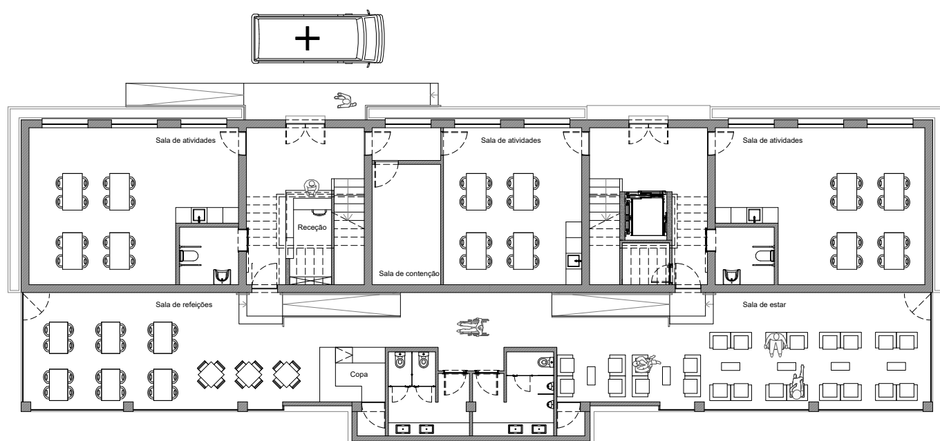
PLANTA PISO 1
